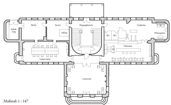
Grundriss Schloss Untergeschoss
